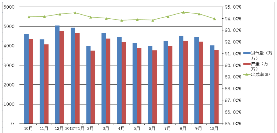
2017年10月——2018年10月吉木乃LNG工厂产量统计图
