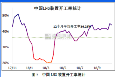
图7 中国LNG装置开工率统计
